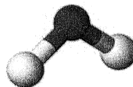
Bent
