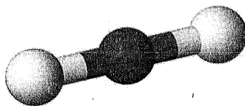
Linear
